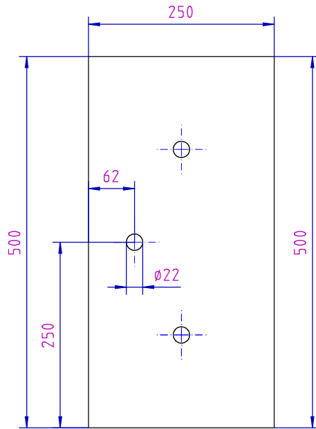
Ansicht ohne Gewindebolzen gezeichnet
